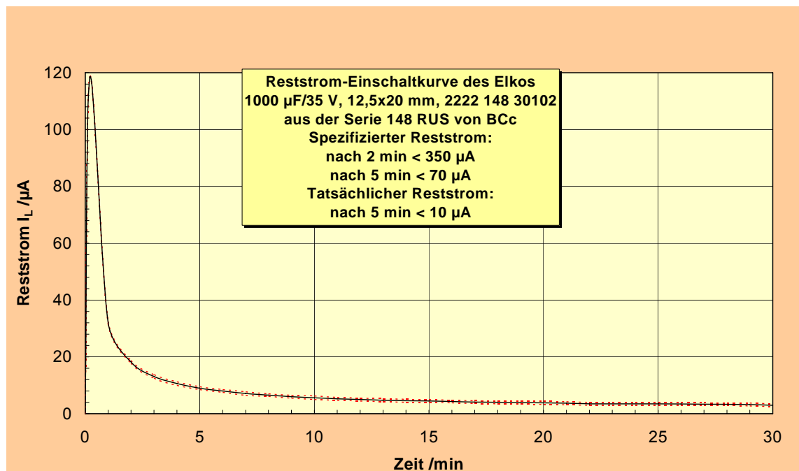
Bild 3 Typischer zeitlicher Verlauf des Reststromes eines Al-Elkos nach dem Einschalten
