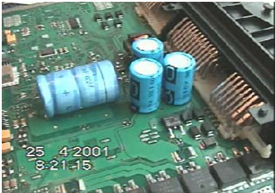
Bild 10 Elektrolytkondensatoren in einer Kfz-Einspritzschaltung von Bosch
