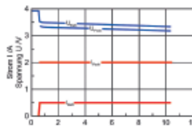
Während des typischen GSM-Betriebes liefert die Batterie einen Strom von 500 mA, mit Peaks von 2 A während der Time-slots, 577 \mu S alle 4,615 ms. Die Kurven UBatt und UPeak zeigen die entsprechende Batteriespannung.
