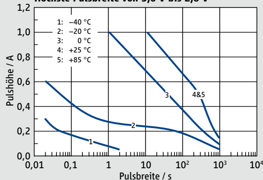
Höchste Pulsbreite von 3,6 V bis 2,8 V
