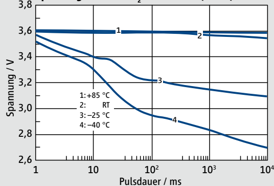
Spannung bei Li/SOCl 2 -Potential (3,67 V), 350 mA
