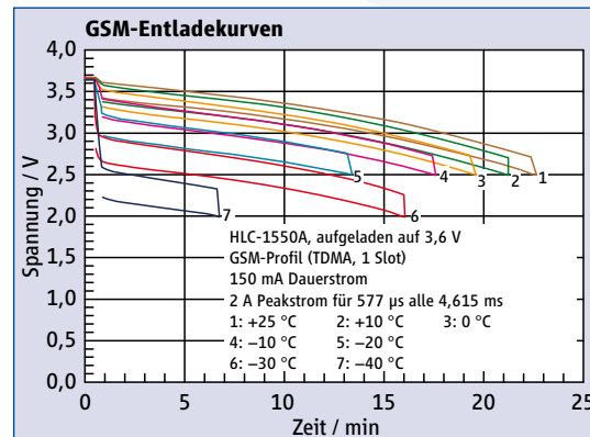
Abb. 2: GSM-Entladekurven
