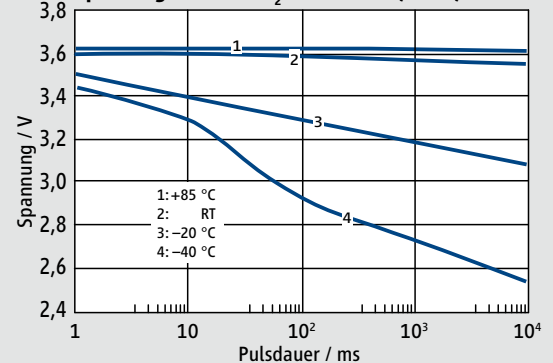
Spannung bei Li/SOCl 2 -Potenzial (3,67 V), 100 mA
