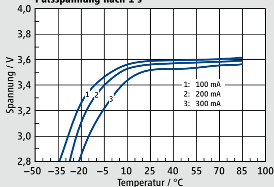
Pulsspannung nach 1 s
