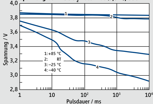
Spannung bei Li/SOCl 2 -Potential (3,9 V), 350 mA
