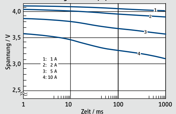
Pulsstromfähigkeit bei RT, 4,2 V Potenzial
