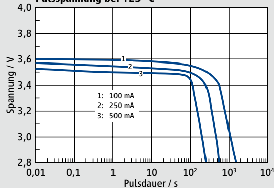
Pulsspannung bei +25 °C
