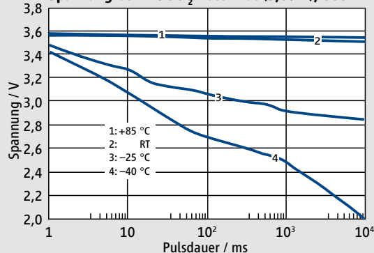
Spannung bei Li/SOCl 2 -Potential (3,67 V), 600 mA
