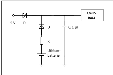
Abbildung 7-1 Grundsaltung zur Batteriepufferung mit Sicherheitselementen (Dioden und Widerstand) gemäß Fall B der UL-Empfehlung. Im Fall A wird der Widerstand R durch eine weitere Diode ersetzt.
