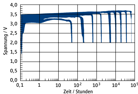
Abbildung 2-9 Datenbank für die Entladung von 1/2AA-Zellen des Typs SL-350 bei +25 °C
