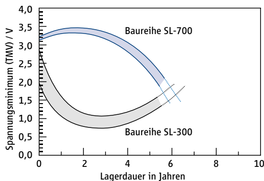
Abbildung 2-4 Typisches Verhalten des Spannungssackes als Funktion der Lagerdauer für zwei Baureihen Entladung bei 25 °C mit 100-stündigem Strom (2 mA/cm 2 )
