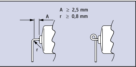
Abbildung 8-1 kleinste Biegemasse für Drahtanschlüsse, alternative Anordnung
