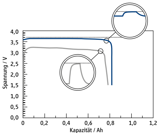
Abbildung 2-1 Entladekurven von Zellen der Größe 1/2AA, Typ SL-350, bei +25 °C graue Kurve: 180 \Omega (30 Stunden) blaue Kurve: 180 k \Omega (4 Jahre) Die Kreise deuten die Erholung der Spannung auf 3,67 Volt an (unterbrochene Linie), immer wenn die Entladung unterbrochen wird.
