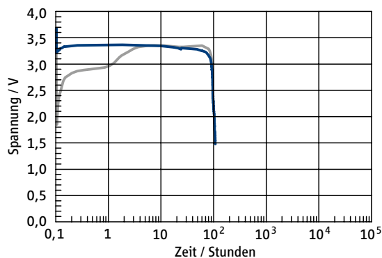
Abbildung 2-3 Entladung von \frac{1}{2} AA-Zellen an 330 \Omega nach einem Jahr Lagerung bei +25 °C
