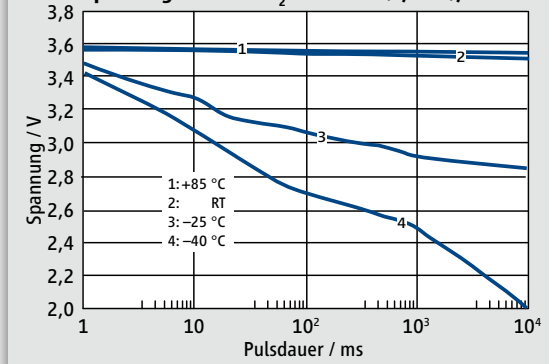
Spannung bei Li/SOCl 2 -Potenzial (3,67 V), 1200 mA
