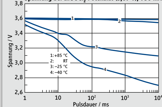
Spannung bei Li/SOCl 2 -Potenzial (3,67 V), 750 mA
