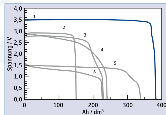
Abb. 2: Vergleich verschiedener Batteriesysteme. Die Kurven stellen die typischen Bestwerte handelsüblicher Rundzellen dar. Entladebedingung 25 °C bei 1000-stündigem Strom. Die Fläche unter den Kurven entspricht der in der Liste unten angegebenen Energiedichte.
