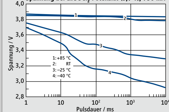
Spannung bei Li/SOCl 2 -Potenzial (3,9 V), 750 mA
