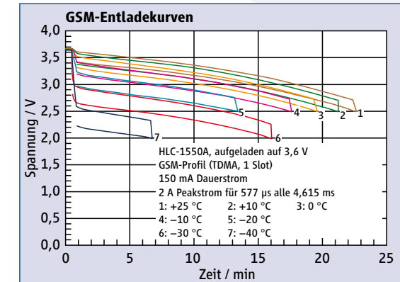
Abb. 2: GSM-Entladekurven
