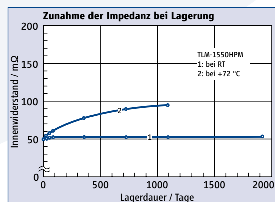
Abb. 3: Zunahme der Impedanz bei Lagerung
