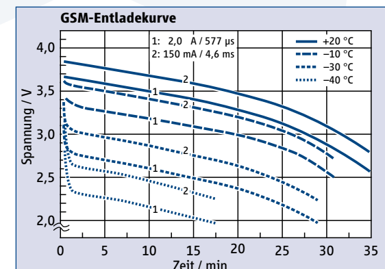
Abb. 2: Entladekurve der TLI-1550A unter einem GSM-Lastprofil nach einer Lagerung für einen Monat bei 72 °C. Die Last wird fortwährend zwischen den beiden Betriebszuständen gewechselt.
