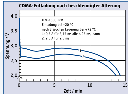
Abb. 2: CDMA-Entladung nach beschleunigter Alterung
