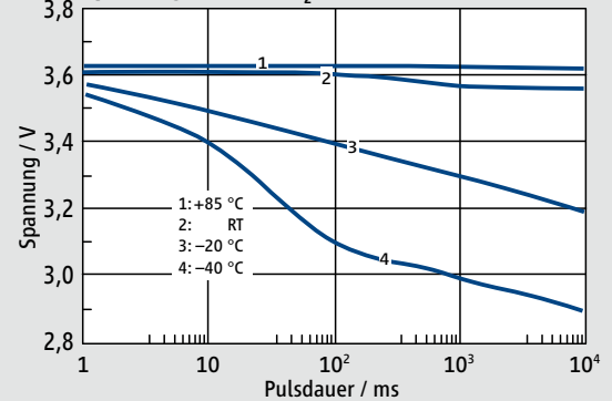
Spannung bei Li/SOCl 2 -Potenzial (3,67 V), 60 mA
