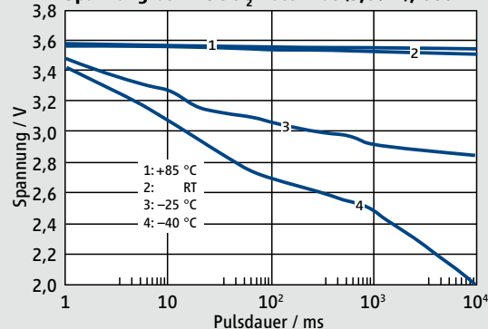
Spannung bei Li/SOCl 2 -Potenzial (3,67 V), 600 mA
