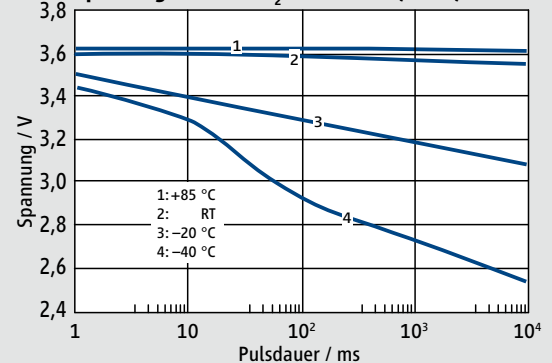
Spannung bei Li/SOCl 2 -Potenzial (3,67 V), 100 mA
