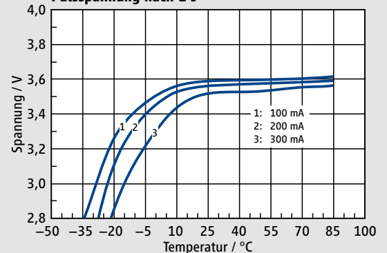
Pulsspannung nach 1 s
