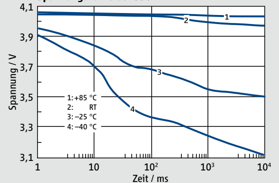
Spannungskurve bei 750 mA
