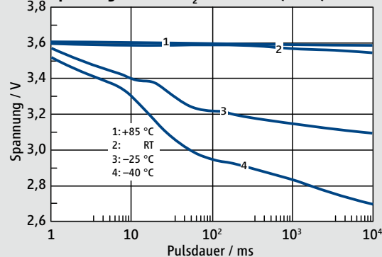
Spannung bei Li/SOCl 2 -Potenzial (3,67 V), 350 mA
