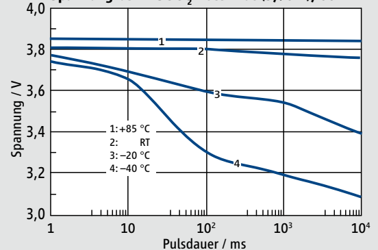
Spannung bei Li/SOCl 2 -Potenzial (3,90 V), 60 mA
