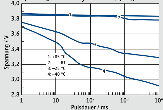
Spannung bei Li/SOCl 2 -Potenzial (3,9 V), 350 mA
